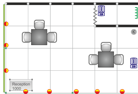
Пример планировки 24 кв.м
